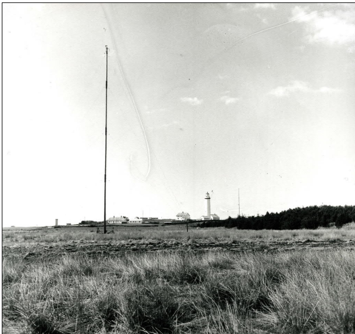
LKE Lista Kringkaster. Sendermast nær Lista fyr. I bakgrunnen T-antenne (sendermast-fyrtårn) for radiofyret "LA", 296,5, så 300,5 kHz, senere ombygd til DGPS-sender.) Bilde©Fædrelandsvennen, Kristiansand S(080574?)
