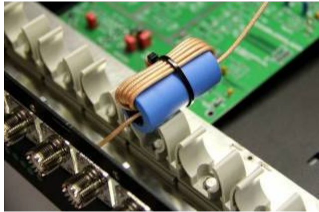
Första common mode choken på plats
