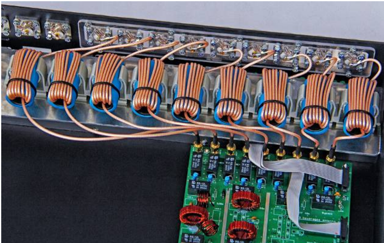
Alla common mode chokes på plats och inkommande antennanslutningarna är kopplade till kretskortet.
