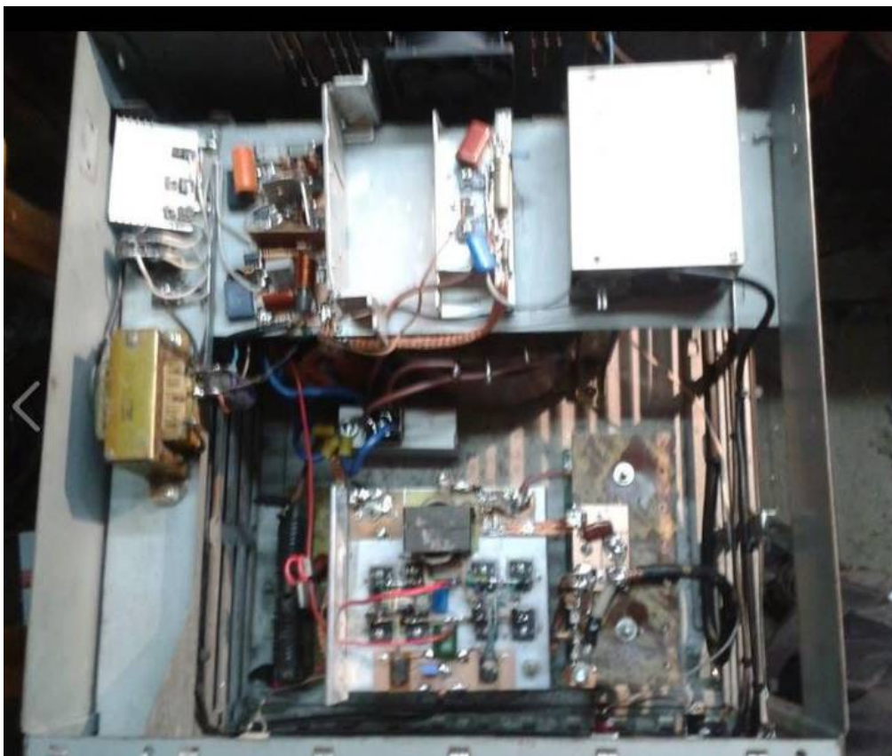
Radio Santa Fé, ARG: Bild på del av AM modulatore. Byggt av Gustavo Halcon, bild från hans Facebooksida
