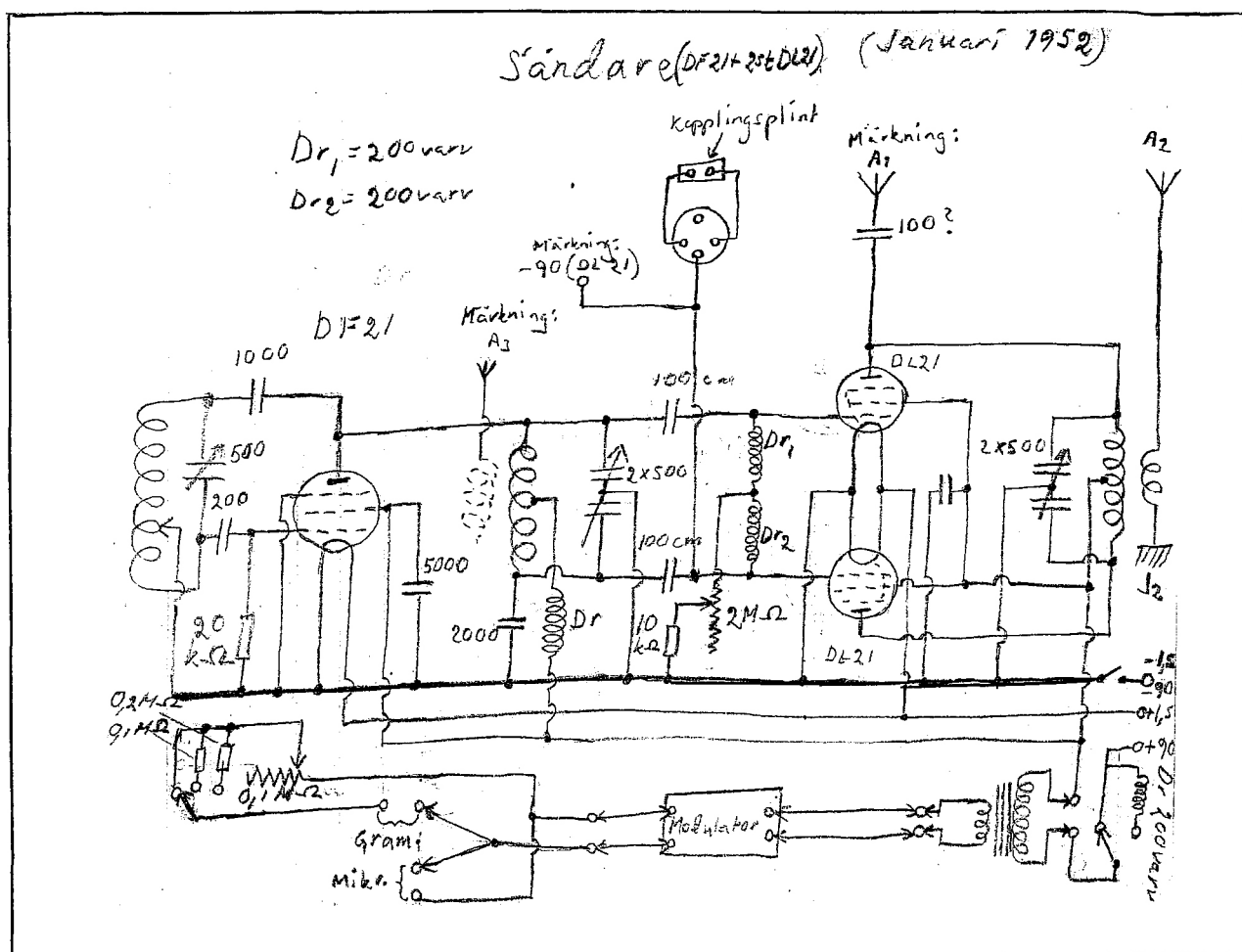
Figur 3. Sändarens kopplingsschema, daterat januari 1952. Jag har inte noterat varifrån jag hämtat schemat, men vid denna tid var det vanligt att hitta sådana i både svensk och utländsk radiopress.
