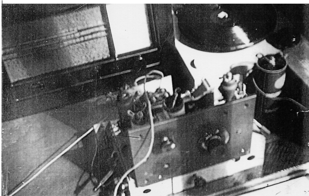
Figur 2. Sändarens huvudkomponenter: Radiolan = modulatorn, skivspelaren, sändaren och batterier (delvis skymda), som framgår av texten samt av schemat figur 3.
