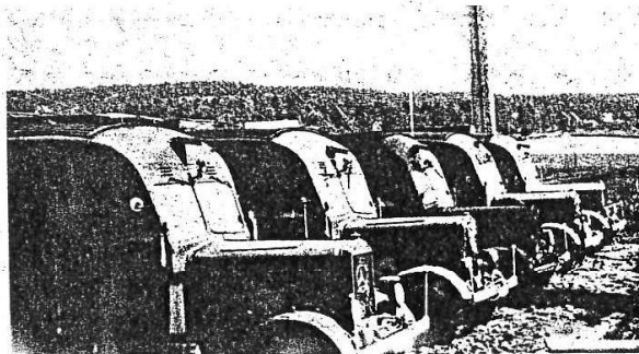
Nedan: Den transportabla sändaren uppställd för sändning. (Den sjätte bilen är antennvagnen på bilden längst t. h.)
